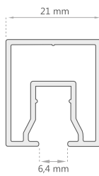
Marco Fijo Corto K-0304/6
