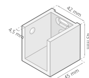
SOPORTE GUÍA DERECHO
