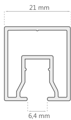
Marco Fijo Cierre Corto K-0304/6
