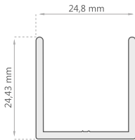
Marco Fijo Corto K-0304
