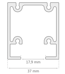
Guía Superior 2 Hojas Correderas D-2116
