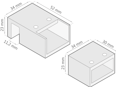
Conjunto Soporte Vidrio Tubo
