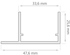
Expansor D-2112
