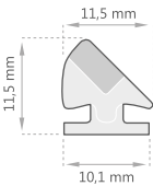
Imán Enfundado C-0844
