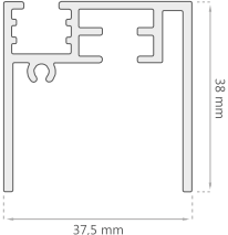
Guía Superior Cerrada D-2096
