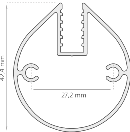
Tubo Autorretornable D-2034
