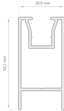
Marco Fijo D-2029
