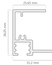
Esquinero F.L. D-2102
