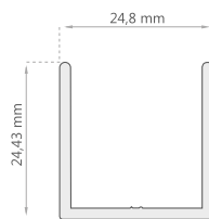
Marco Fijo Corto K-0304/6
