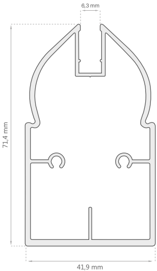
Marco Fijo D-2013
