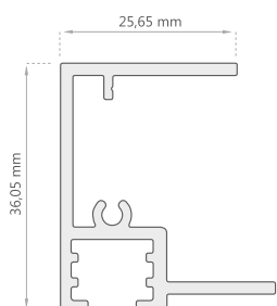
Esquinero F.L. D-2102
