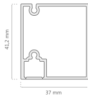
Marco esquinero D-2108
