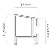
Perfil Base D-2091
