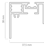
Guía Superior D-2075
