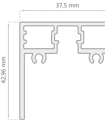
Marco Lateral 2 Hojas Correderas D-2117
