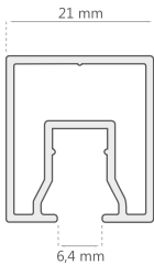
Marco Fijo Corto K-0304
