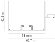
Guía Superior D-2065
