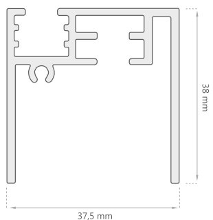
Esquinero F.L. D-2102
