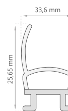
Junquillo Estanqueidad Pivotante PGE-1438
