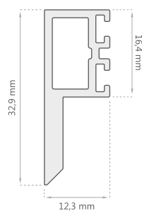
Expansor Marco Fijo Corto J-1110
