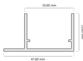
Expansor D-2112
