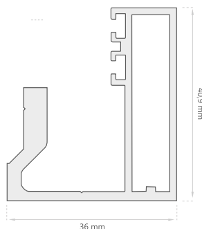
Marco Fijo D-2080
