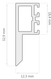
Marco Cierre D-2081
