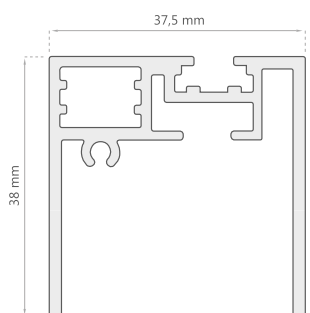
Marco Fijo D-2107
