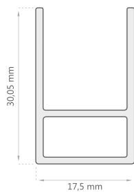
Marco Fijo F.L. Corto K-0304/8
