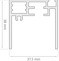
Marco Imán D-2100
