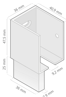
Soporte Guía Pared Izquierdo
