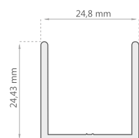
Expansor Marco Fijo Corto J-1110
