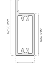
Guía Inferior 2 Hojas Correderas D-2115
