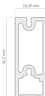
Guía D-2106
