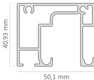
Guía Superior D-2065
