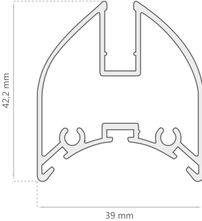
Marco Fijo/Bisagra autorretornable D-2014
