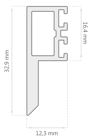
Tapa Marco D-2077
