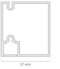
Perfil Superior Lateral Fijo D-2103
