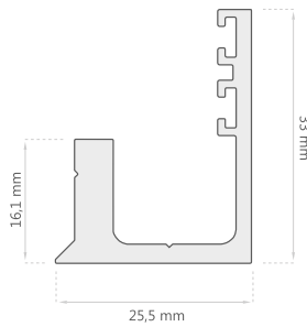
Marco Fijo D-2076
