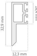
Tapa Marco D-2077
