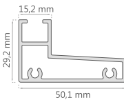
Guía inferior D-2064
