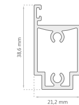
Expansor D-2112
