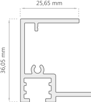
Esquinero F.L. D-2102
