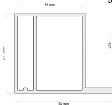
Marco Cierre D-2081
