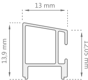
Perfil Base D-2091
