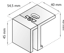
Ángulo Central Reglable
