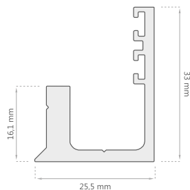
Tapa Marco D-2077
