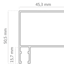
Esquinero F.L. D-2054
